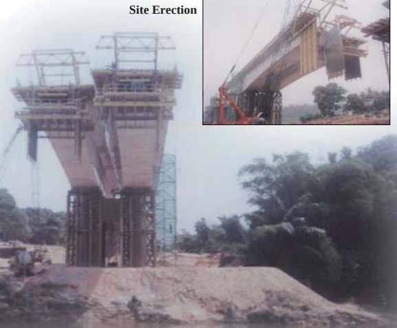
Site Erection
